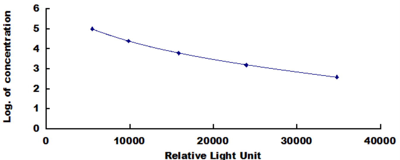
精氨酸(Arg)检测试剂盒标准曲线
