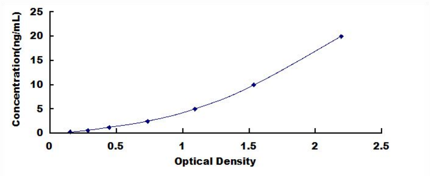
小鼠血管紧张素转化酶(ACE)检测试剂盒标准曲线
