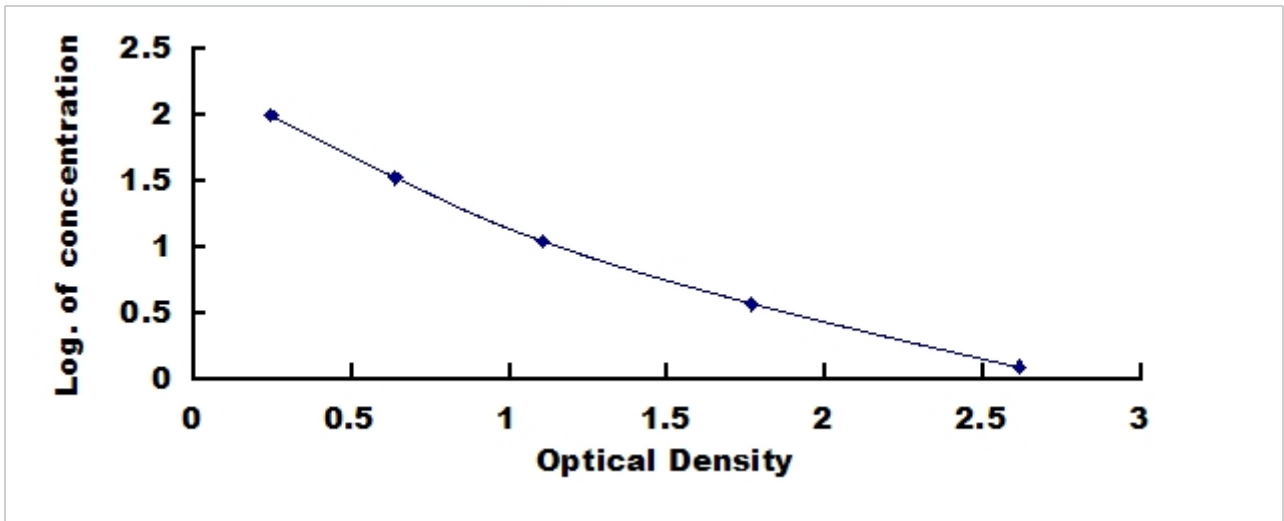
精氨酸 (Arg) 检测试剂盒标准曲线
