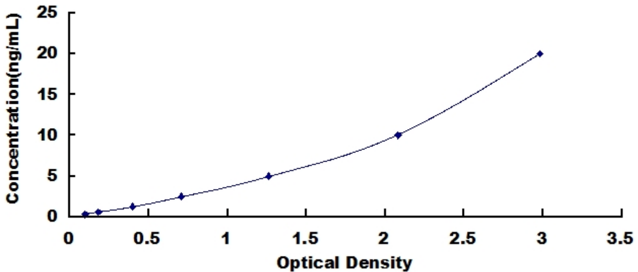
人 B-细胞淋巴瘤因子 2 样蛋白 (Bcl2L) 检测试剂盒标准曲线
