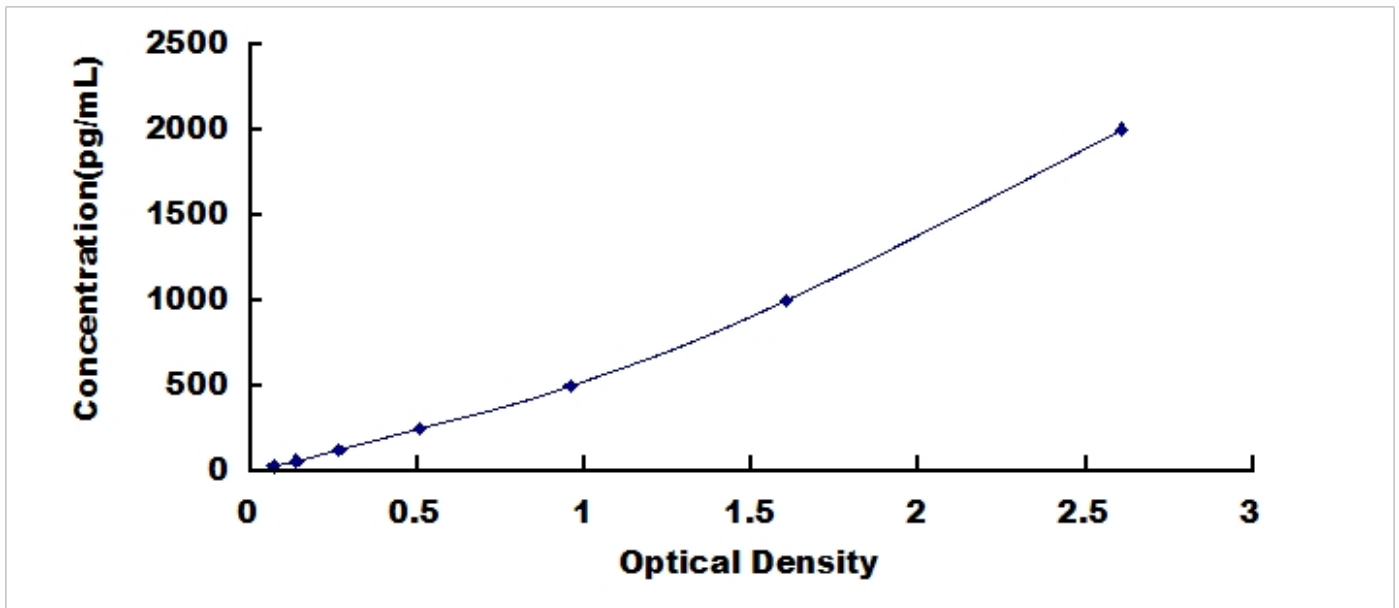
人骨成型蛋白 3 (BMP3) 检测试剂盒标准曲线
