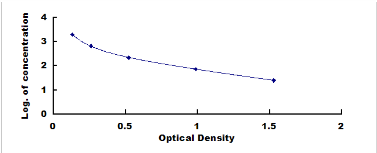
人脑钠素 (BNP) 检测试剂盒标准曲线
