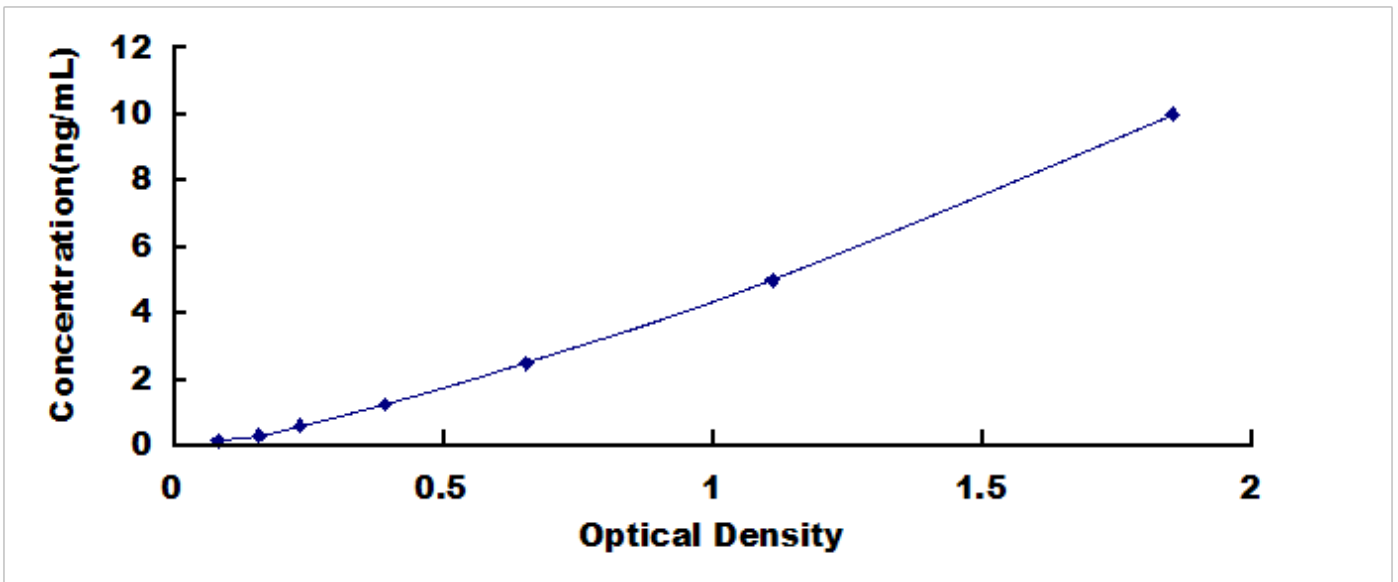
人戴帽蛋白肌 Z 系 \beta (CAPZ \beta ) 检测试剂盒标准曲线
