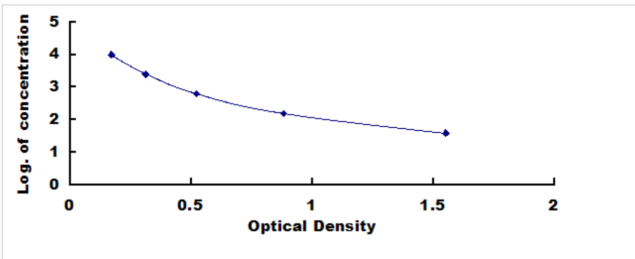
硫酸软骨素 (CS) 检测试剂盒标准曲线
