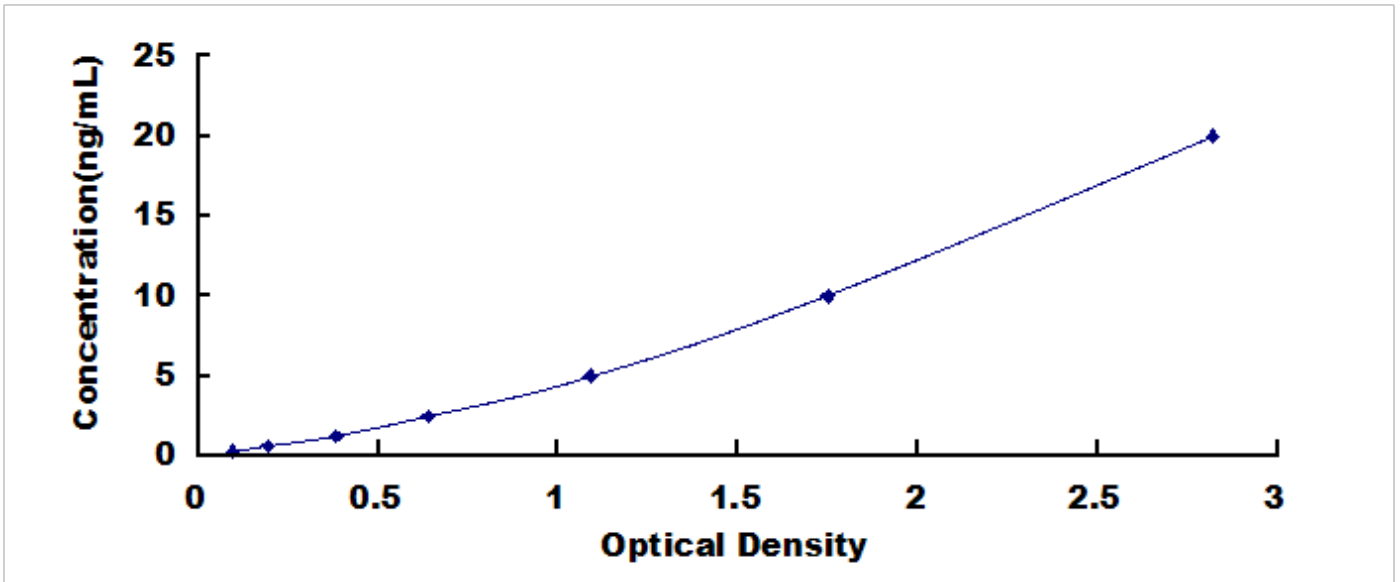
大鼠封闭蛋白 7 (CLDN7) 检测试剂盒标准曲线
