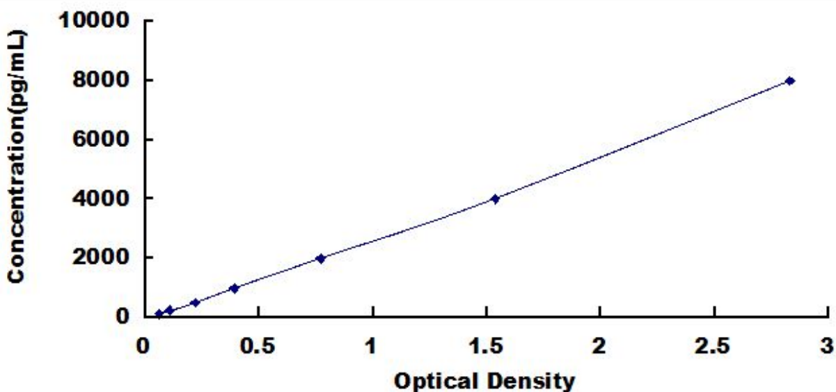
人凝血因子 V (F5) 检测试剂盒标准曲线
