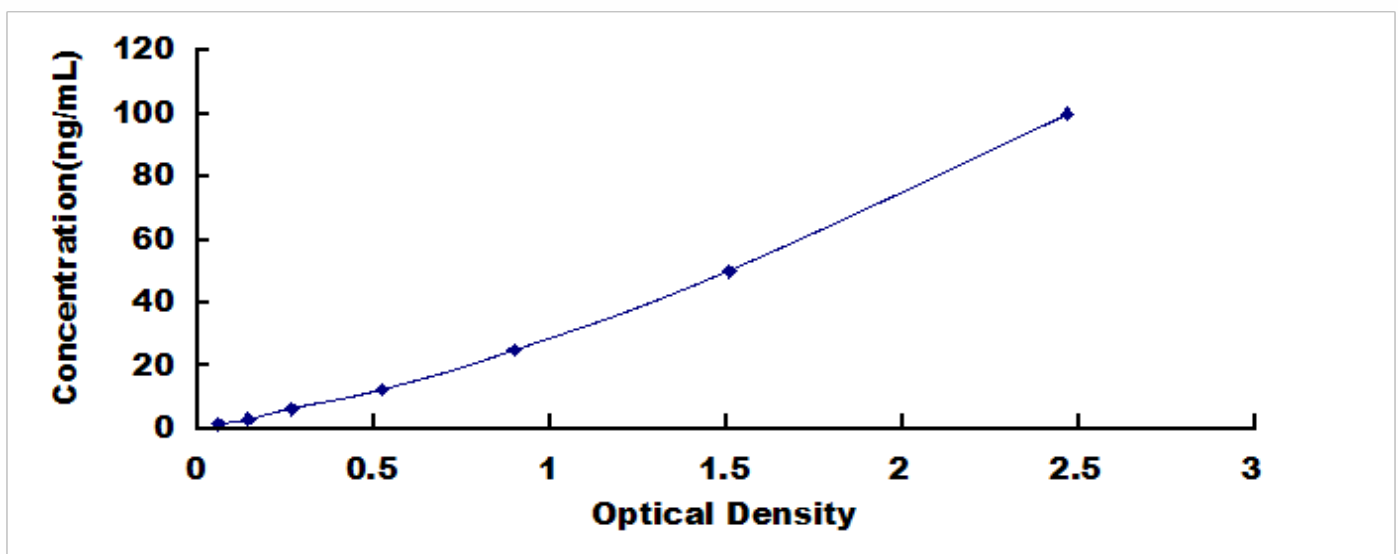
大鼠 I 型胶原 \alpha 2 (COL1 \alpha 2) 检测试剂盒标准曲线
