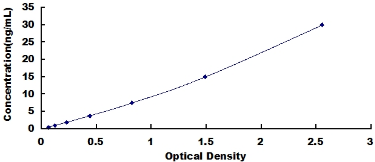
小鼠补体因子 D (CFD) 检测试剂盒标准曲线
