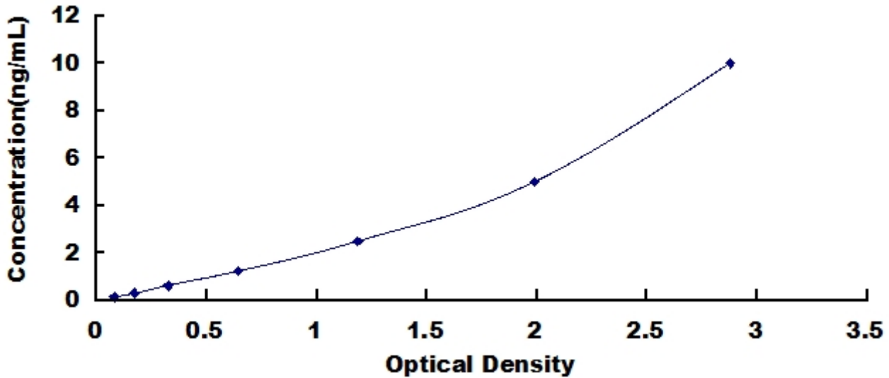
人周期素依赖性激酶 1 (CDK1) 检测试剂盒标准曲线
