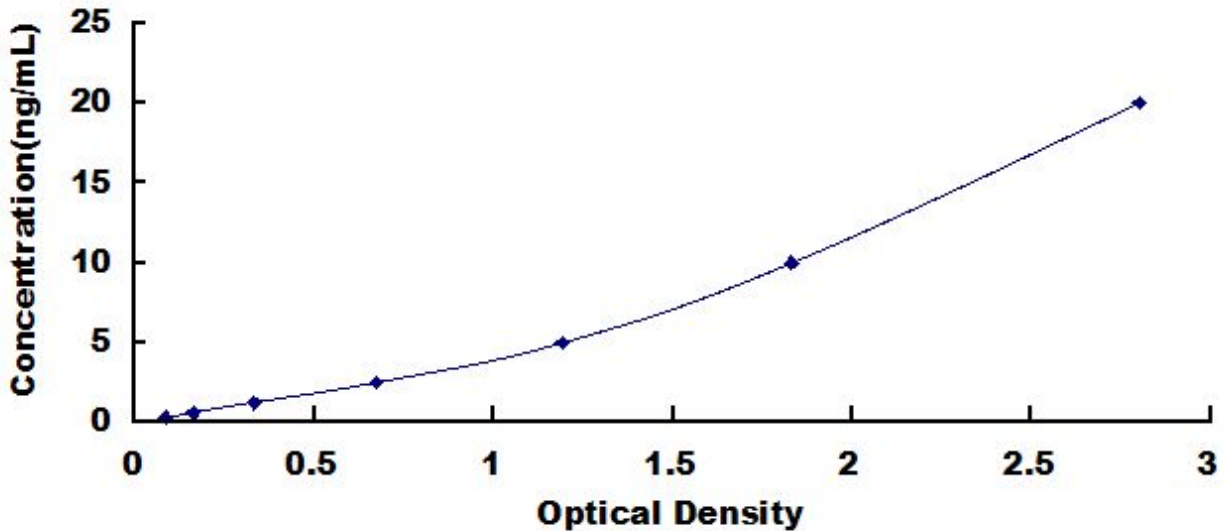
人半胱氨酸丰富跨膜 BMP 调节因子 1 (CRIM1) 检测试剂盒标准曲线
