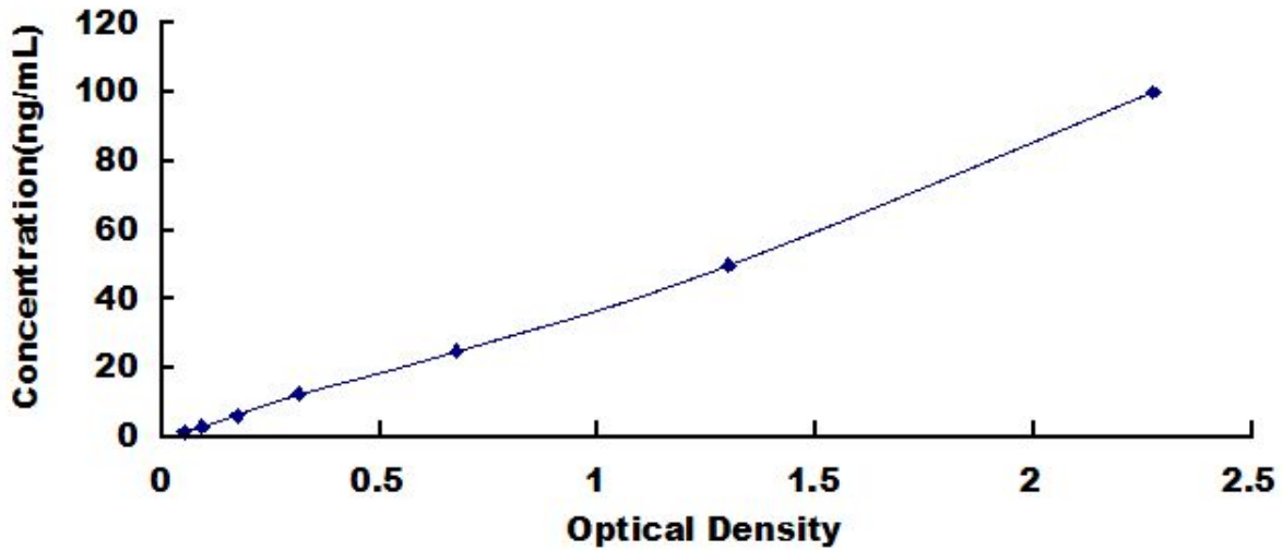
猪防御素 \beta 1 (DEF \beta 1) 检测试剂盒标准曲线
