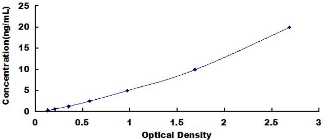
人 EGF 样重复盘状结构 I 样域蛋白 3 (EDIL3) 检测试剂盒标准曲线
