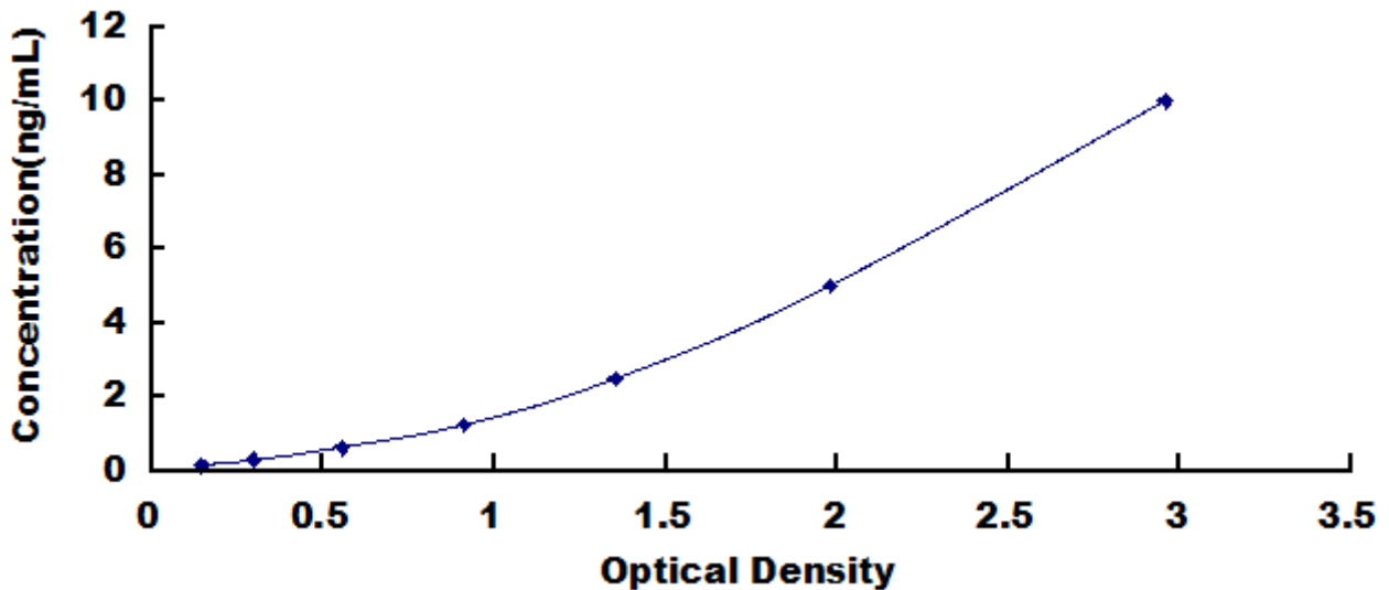
小鼠 FMS 样酪氨酸激酶 3 配体 (F1t3L) 检测试剂盒标准曲线
