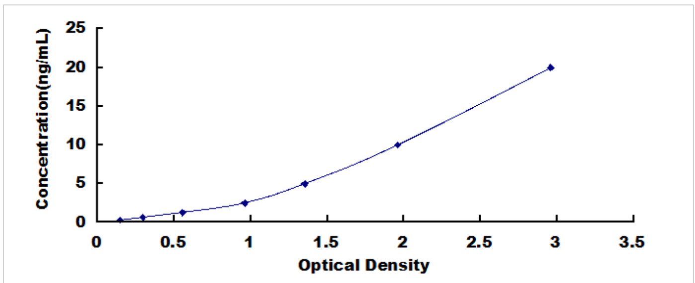
人脂肪酸合酶(FASN)检测试剂盒标准曲线
