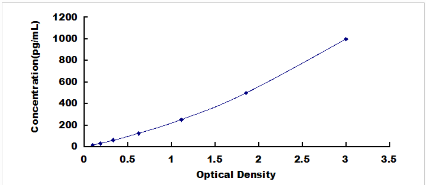
小鼠含III型纤连蛋白域蛋白 5 (FNDC5) 检测试剂盒标准曲线
