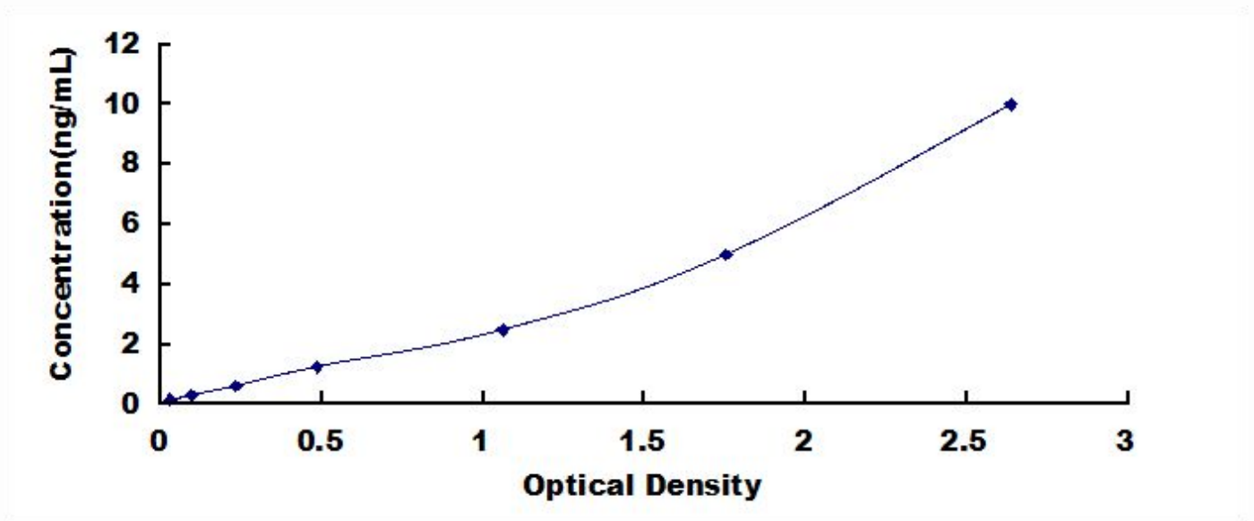
小鼠 G 蛋白 \alpha 激活活性多肽 0 (GNa01) 检测试剂盒标准曲线
