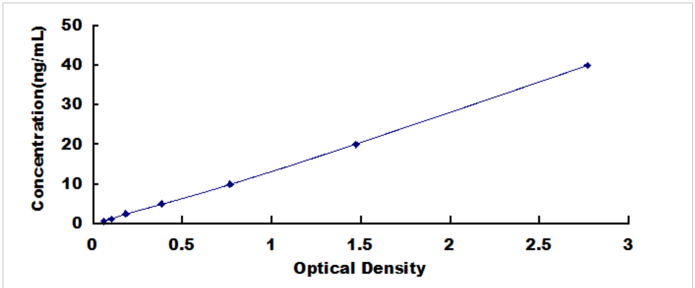
人 G 蛋白偶联受体 120 (GPR120) 检测试剂盒标准曲线
