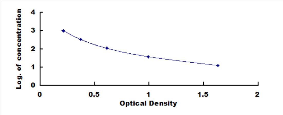
人甘丙肽 (GAL) 检测试剂盒标准曲线
