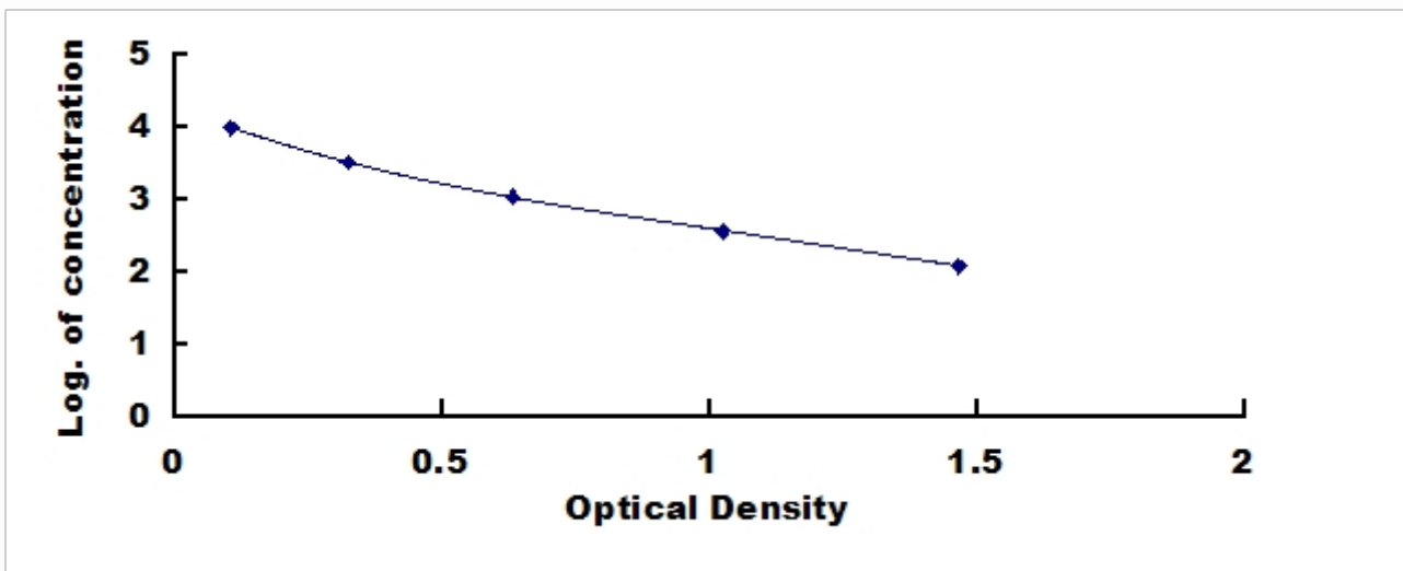
猪饥饿素(GHRL)检测试剂盒标准曲线
