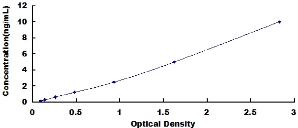
大鼠谷氨酸半胱氨酸连接酶(GCLM)检测试剂盒标准曲线
