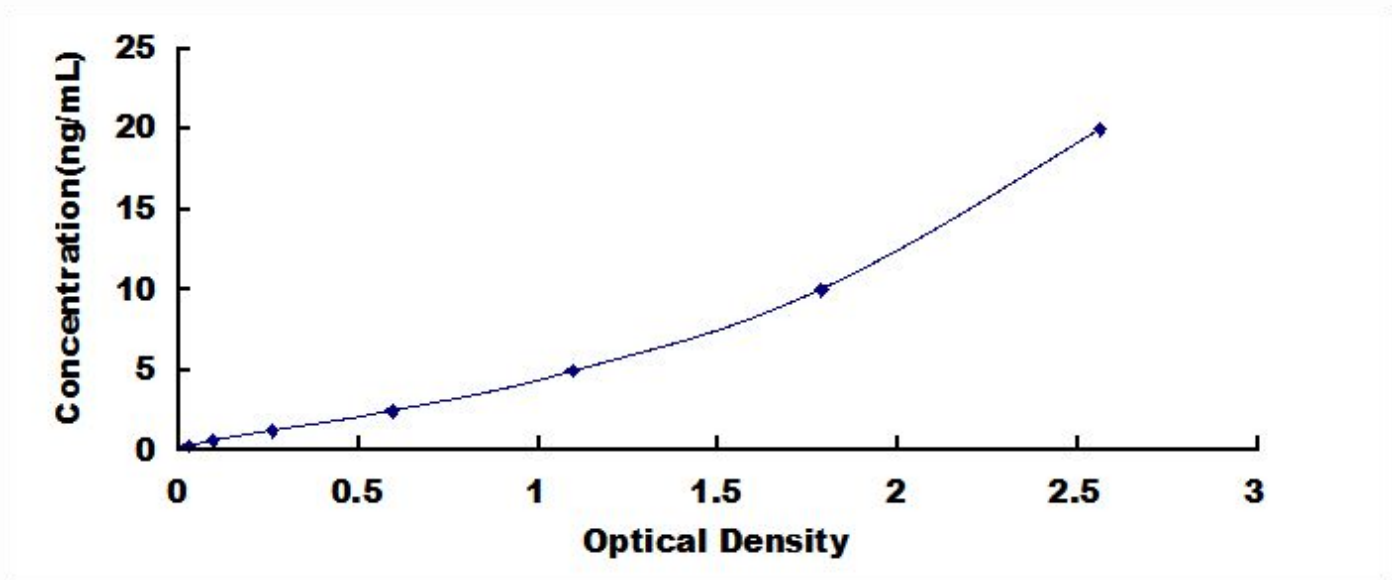
大鼠甘氨酸受体 \alpha 2 (GLR \alpha 2 ) 检测试剂盒标准曲线
