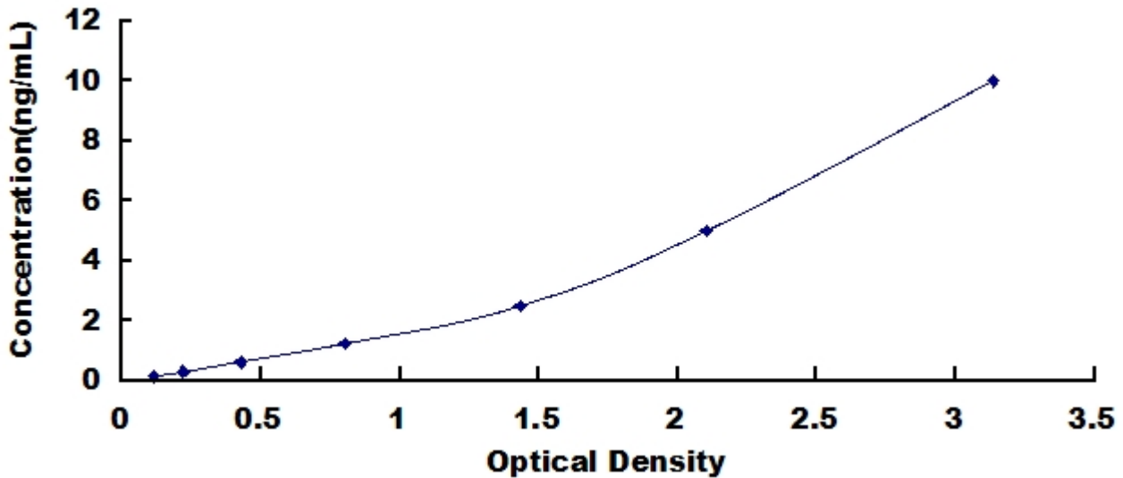
人血小板膜糖蛋白 II b/IIIa (GP II b/IIIa) 检测试剂盒标准曲线
