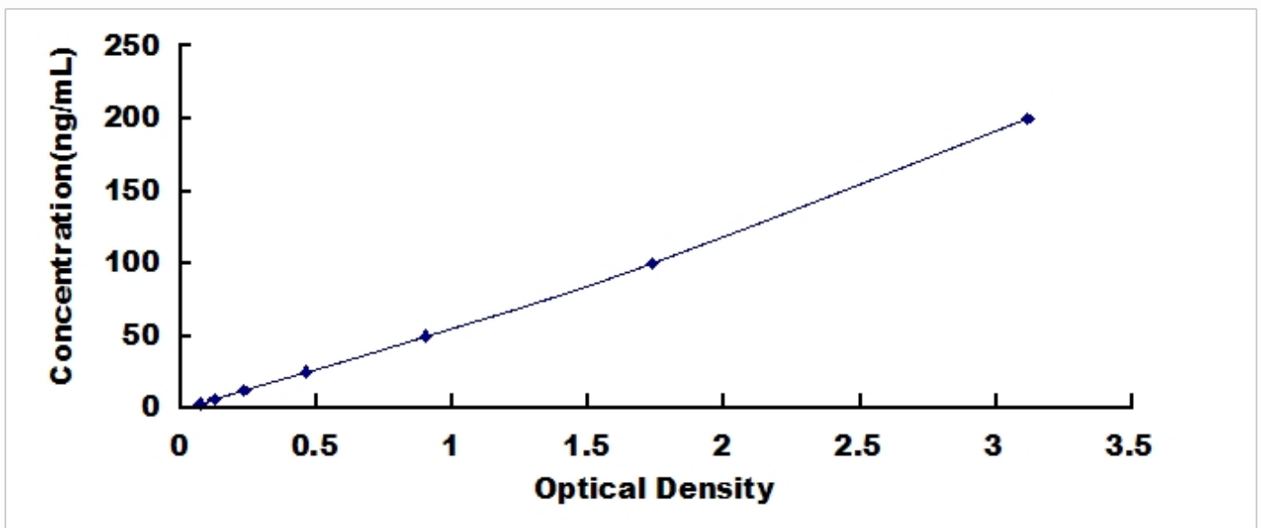
小鼠热休克蛋白 70 (HSP70) 检测试剂盒标准曲线
