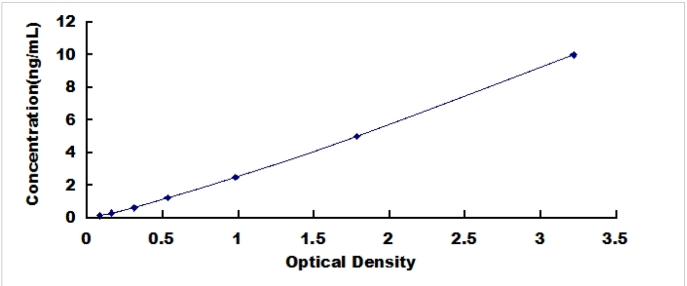
小鼠组蛋白脱乙酰基酶 2 (HDAC2) 检测试剂盒标准曲线
