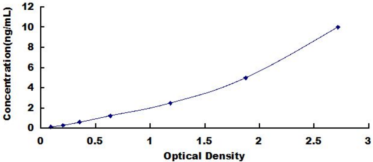
人透明质酸介导运动因子受体(HMMR)检测试剂盒标准曲线
