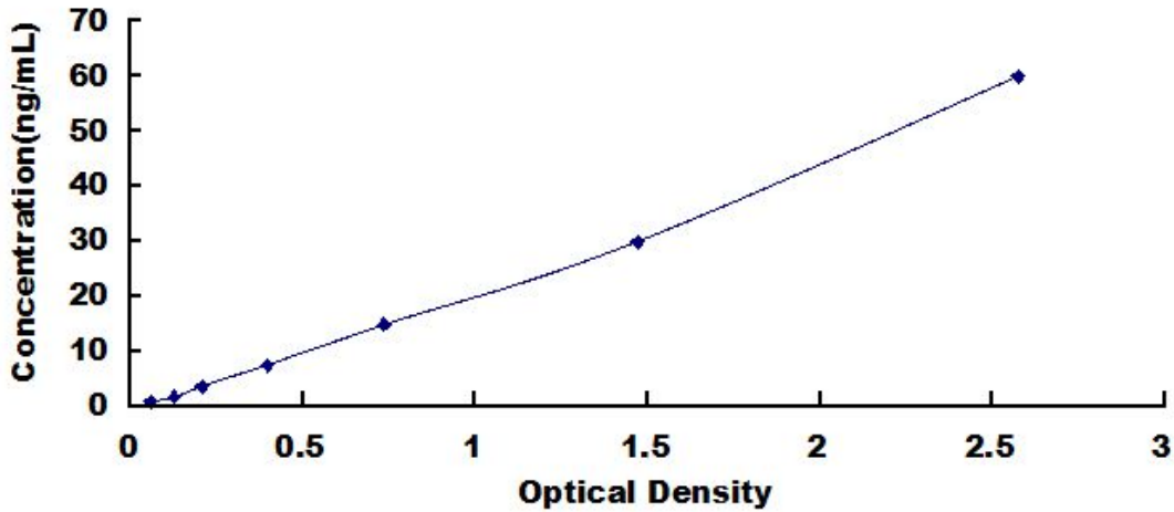
人免疫球蛋白 A2(IgA2)检测试剂盒标准曲线
