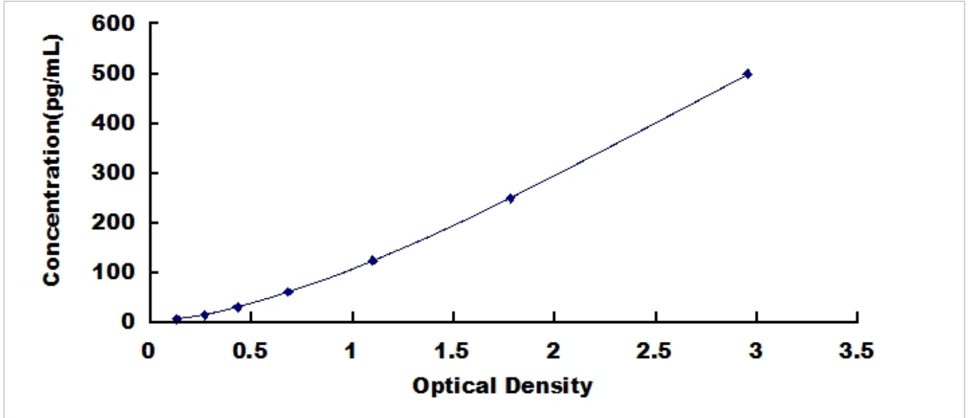
兔白介素 1 受体拮抗剂 (IL1RA) 检测试剂盒标准曲线
