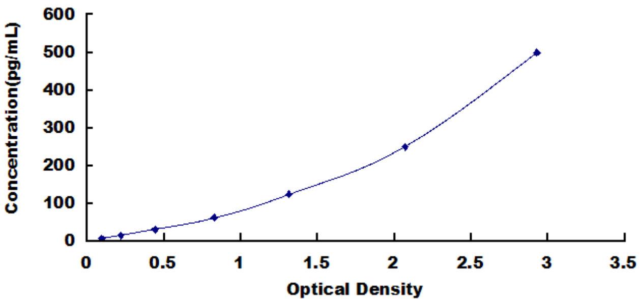
大鼠白介素 10(IL10)检测试剂盒标准曲线
