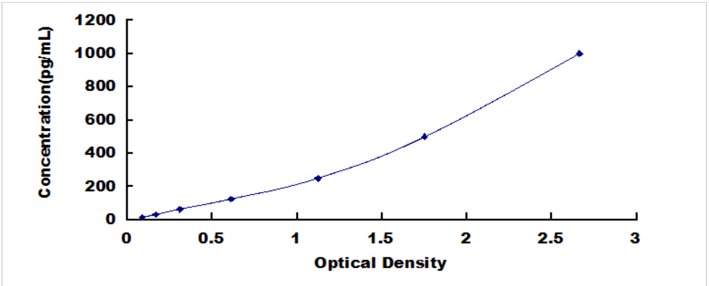
牛白介素 12B (IL12B) 检测试剂盒标准曲线
