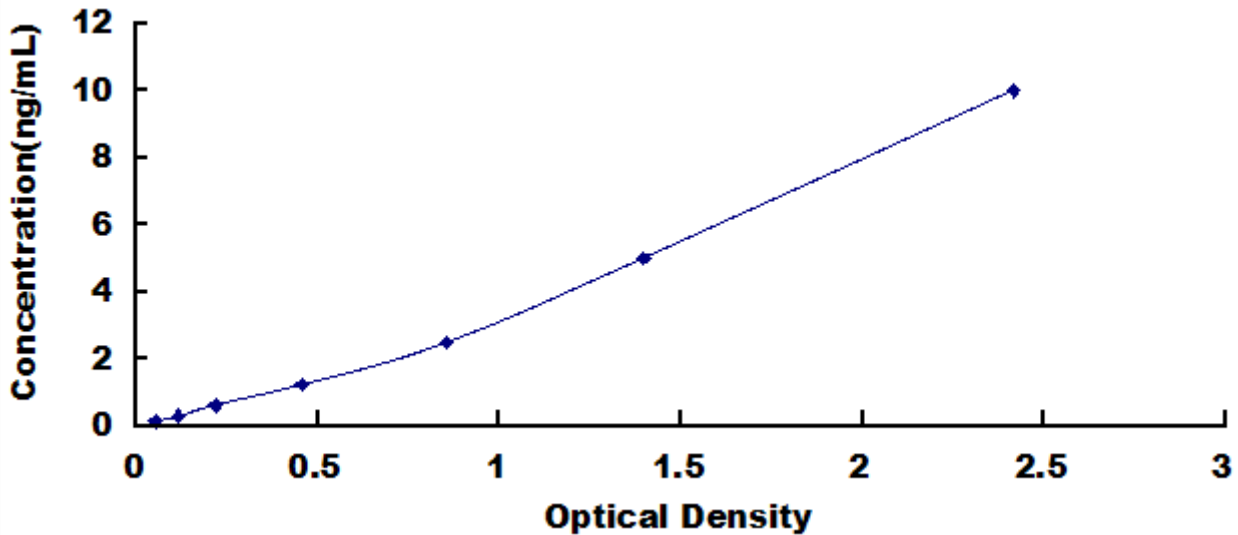
大鼠白介素 8 受体 \alpha (IL8R \alpha ) 检测试剂盒标准曲线
