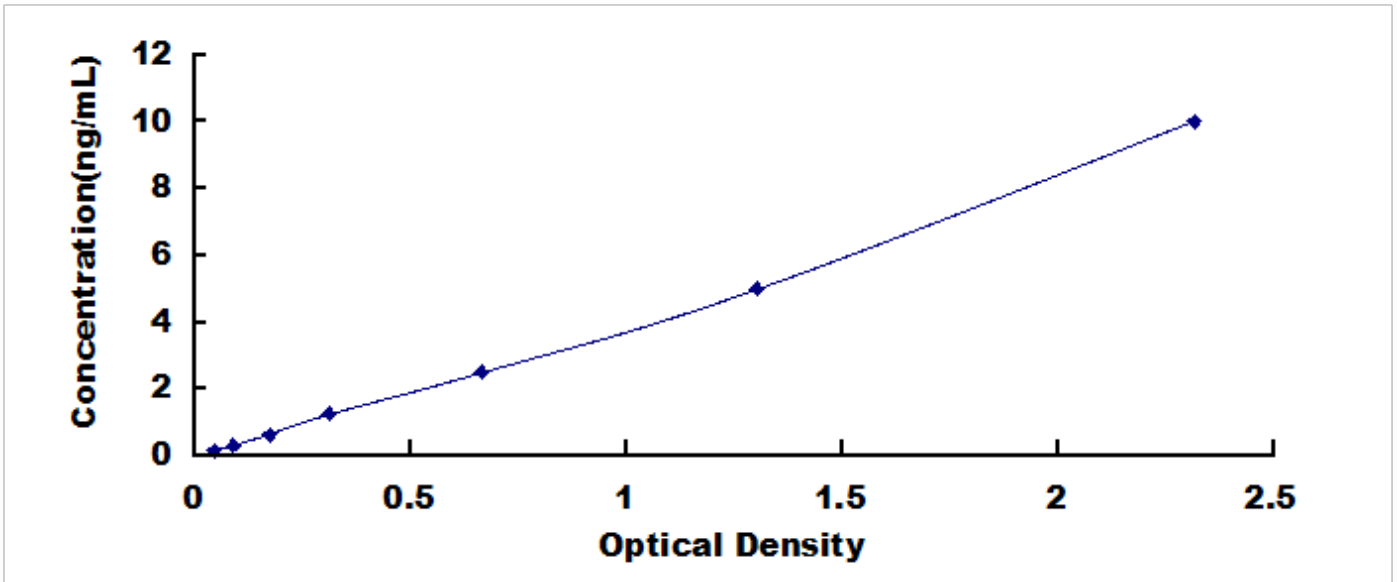
小鼠白介素 8 受体 \alpha (IL8R \alpha ) 检测试剂盒标准曲线
