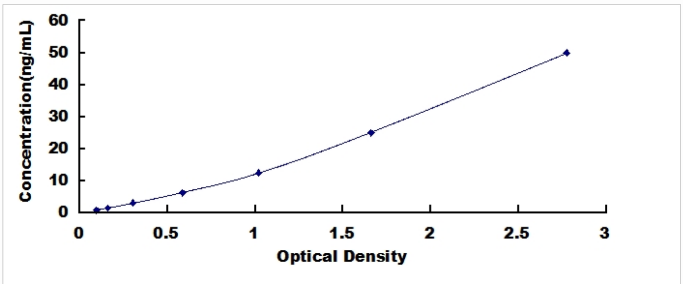
人异柠檬酸脱氢酶 1 (IDH1) 检测试剂盒标准曲线
