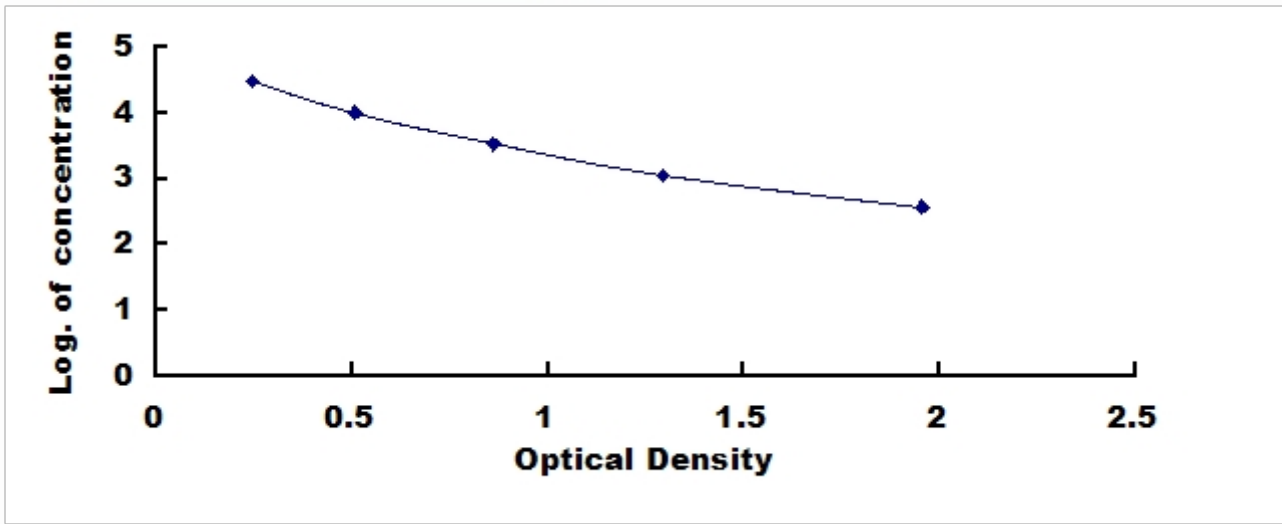
恒河猴黄体激素 (LH) 检测试剂盒标准曲线
