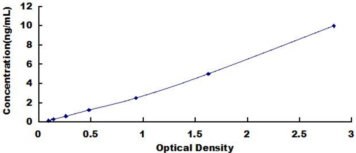
人淋巴增强结合因子 1 (LEF1) 检测试剂盒标准曲线
