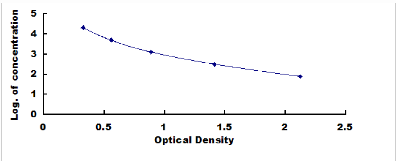
溶血磷脂酰胆碱(LPC)检测试剂盒标准曲线
