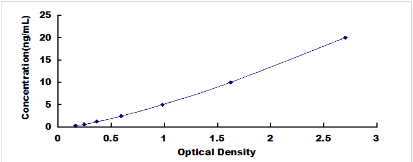
大鼠微管关联蛋白 1 轻链 3 \alpha (MAP1LC3 \alpha ) 检测试剂盒标准曲线
