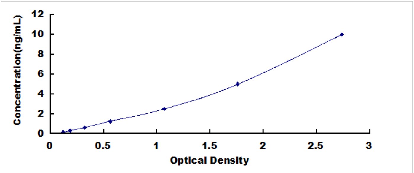
人八聚体结合转录因子 4 (OCT4) 检测试剂盒标准曲线
