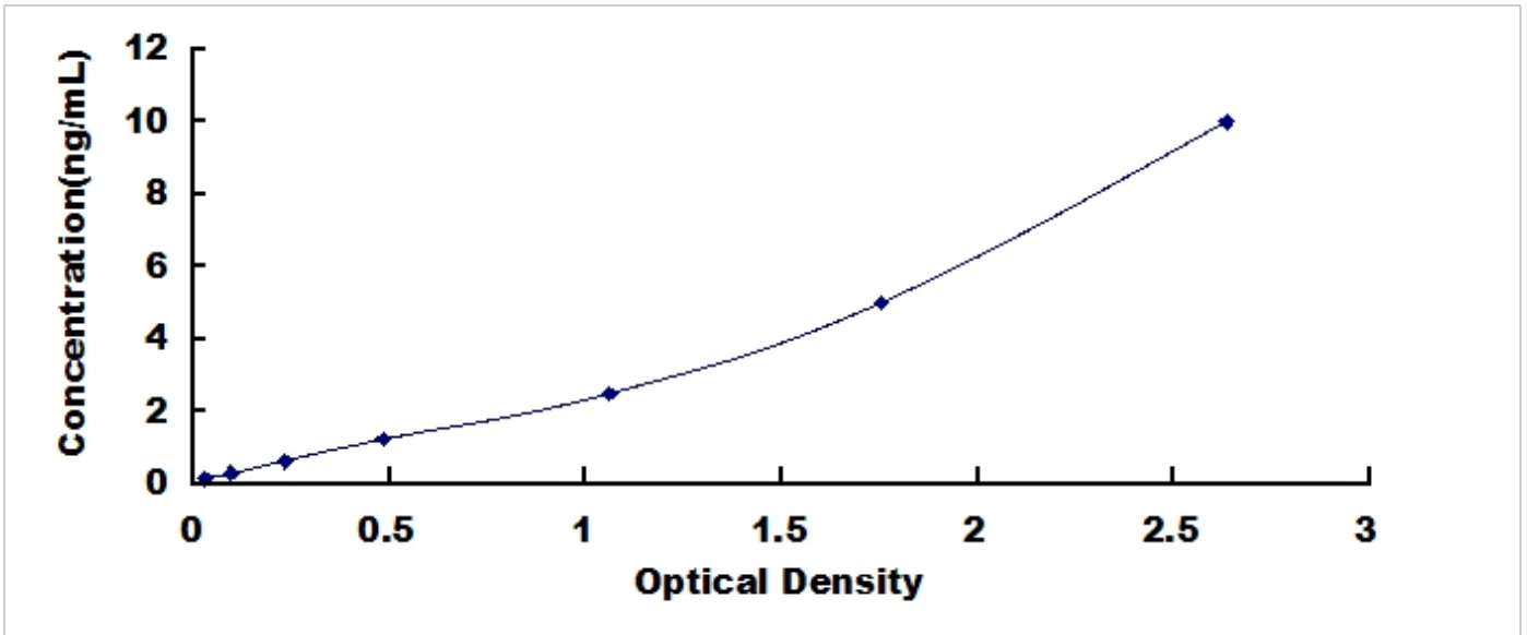
人磷酸肌醇-3-激酶催化亚基 \alpha 肽(PIK3Ca)检测试剂盒标准曲线
