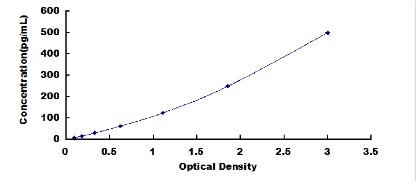
小鼠垂体腺苷酸环化酶激活肽 (ADCYAP1) 检测试剂盒标准曲线
