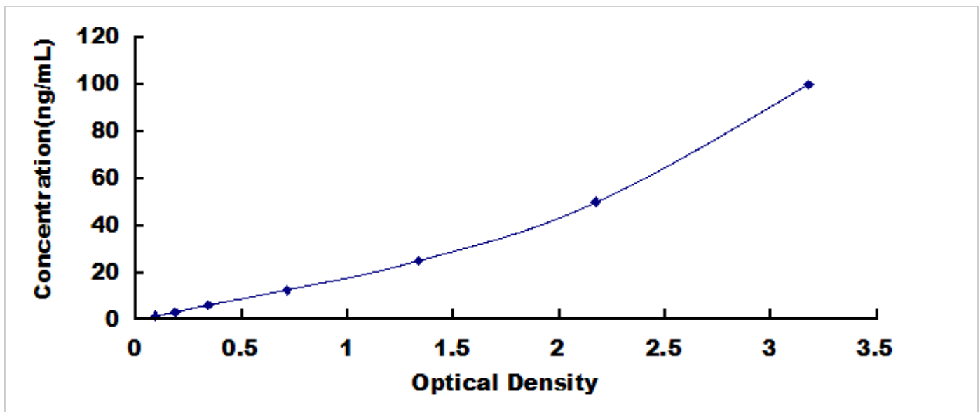
大鼠纤溶酶原激活物抑制因子 2 (PAI2) 检测试剂盒标准曲线
