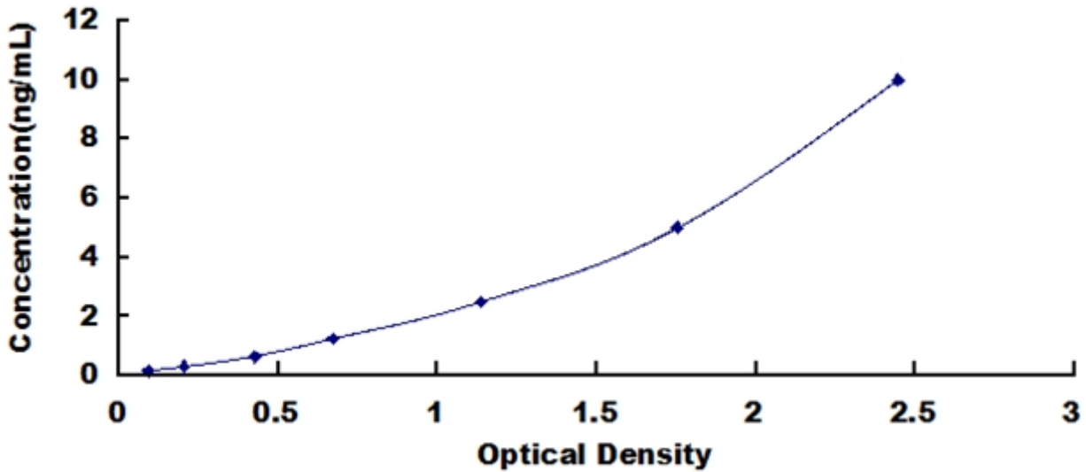
人足孟蛋白 (PODXL) 检测试剂盒标准曲线
