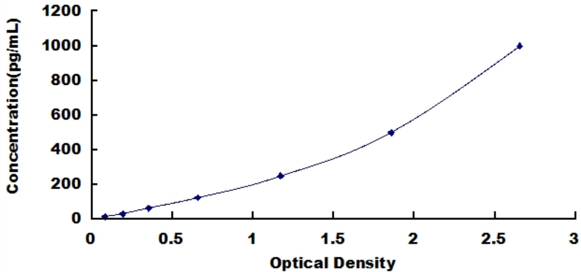
大鼠精氨酸加压素原 (VP) 检测试剂盒标准曲线
