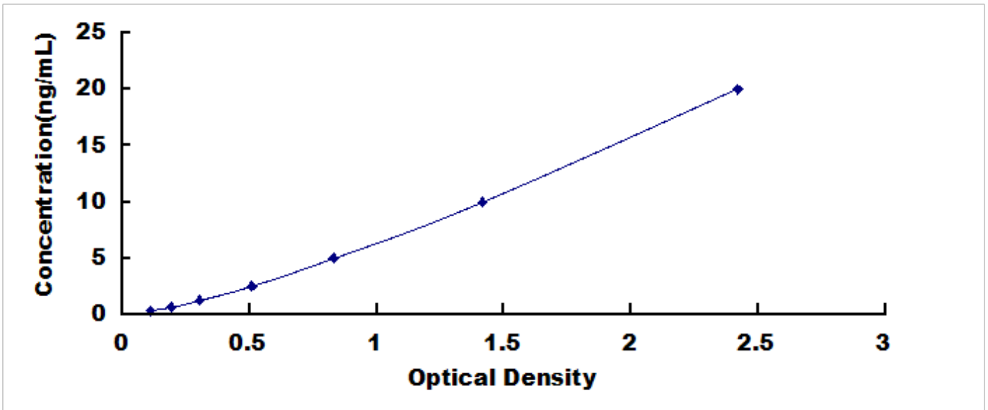
人早老素 1 (PSEN1) 检测试剂盒标准曲线
