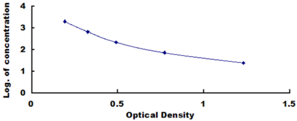
前列环素 (PGI2) 检测试剂盒标准曲线
