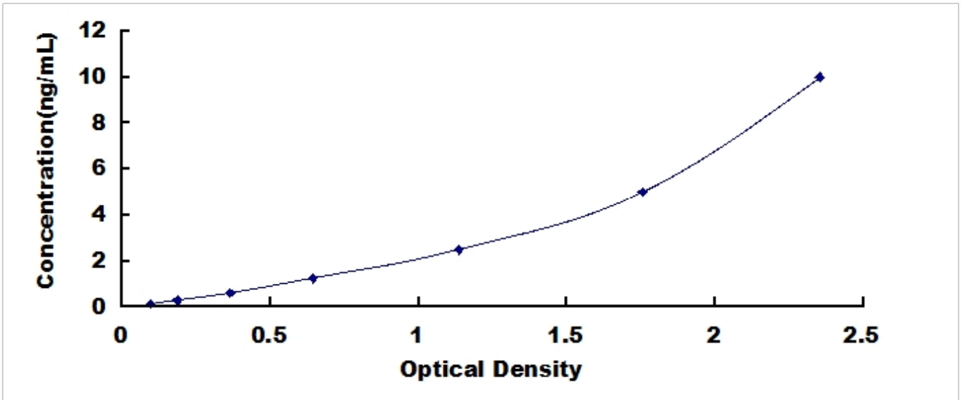
小鼠 cGMP 依赖性蛋白激酶 I (PRKG1) 检测试剂盒标准曲线
