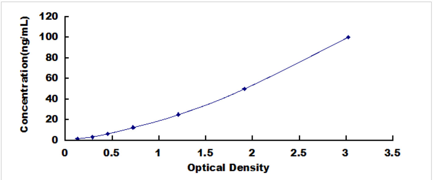
大鼠蛋白激酶 C \zeta (PKC \zeta ) 检测试剂盒标准曲线
